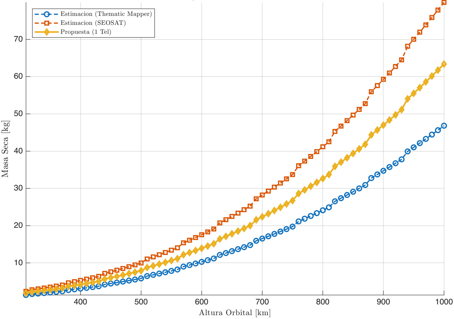
Comparativa de Masa Seca vs. Altura Config: 2 Sat, 1 Tel, Det 1, Korsch
